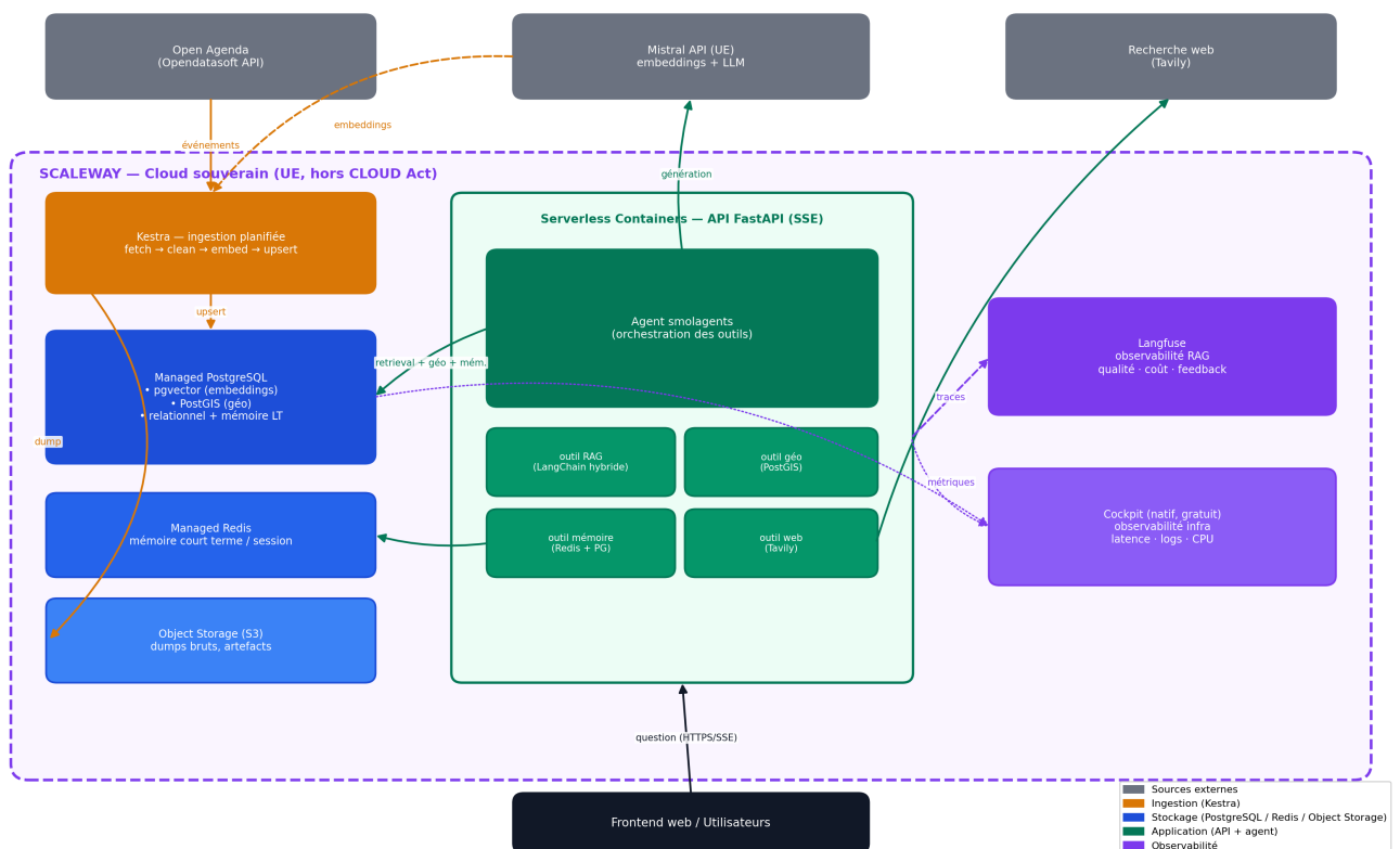
Figure 2 — Déploiement détaillé sur Scaleway (cloud souverain UE, hors CLOUD Act) : ingestion Kestra, base PostgreSQL consolidée, agent smolagents et double observabilité Langfuse + Cockpit.
